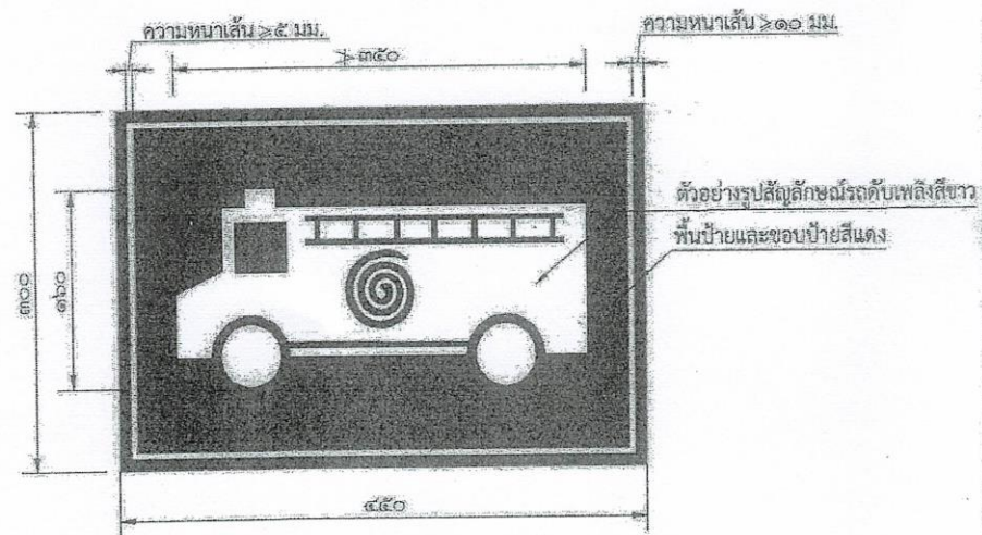
รูปที่ ๑ ขนาด ระยะ รูปแบบป้ายแสดงตำแหน่งพื้นที่สำหรับรถดับเพลิง
